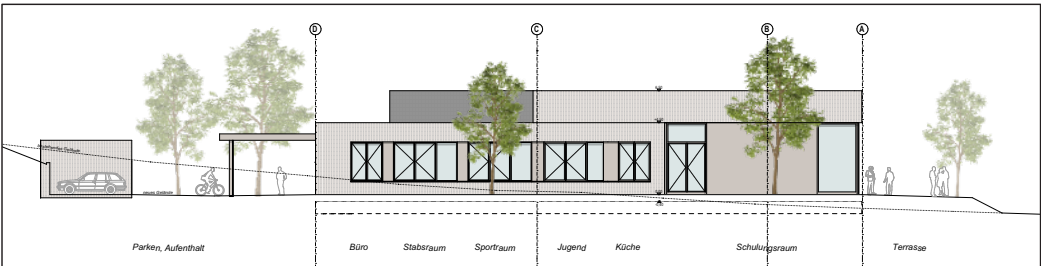
Diesen Entwurf für das künftige Feuerwehrhaus Langensteinbach stellten die Planer im Karlsbader Gemeinderat vor. Zeichnung: Planungsbüro buerohauser
